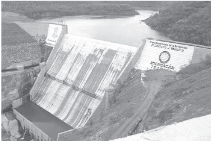
La obra ejecutada por la empresa brasileña Odebrecht, se resquebraja y ha generado una enorme grieta que llegó a la Autopista en el km 148+460.
